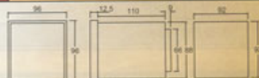
MODEL : 96R-3600, 96R3501-V34, 96R-3501-A34, 96R3501-V33 PANEL CUT-OUT
